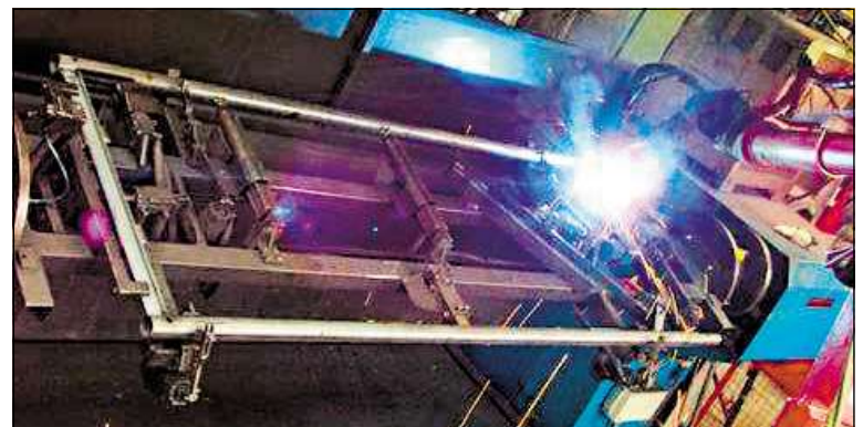
Wiederkehr-System-Gerüste werden in der Schweiz produziert. Hier der Schweisroboter in Aktion...
